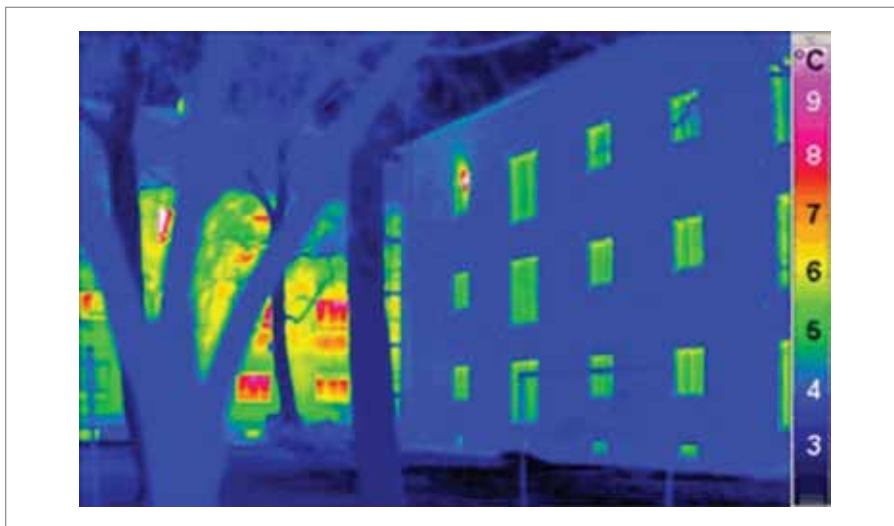
Рис. 5.9 Тепловизионная съемка «пассивно- го» дома (справа) и обычного дома (слева)
